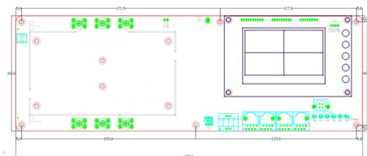
图 10-3 主板尺寸图
