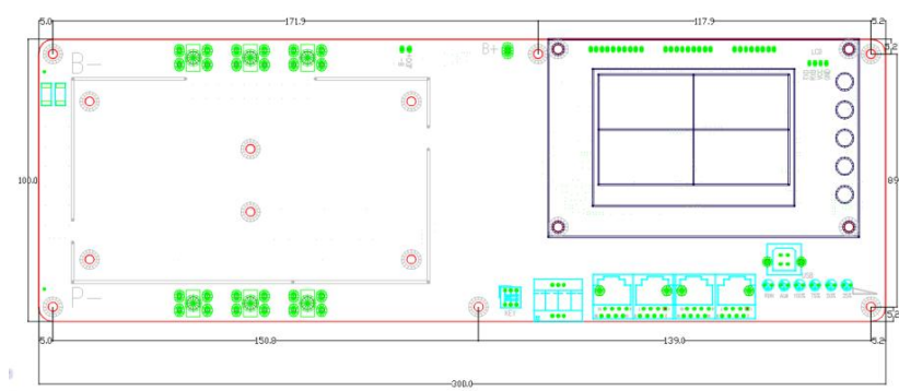
图 10-3 主板尺寸图
