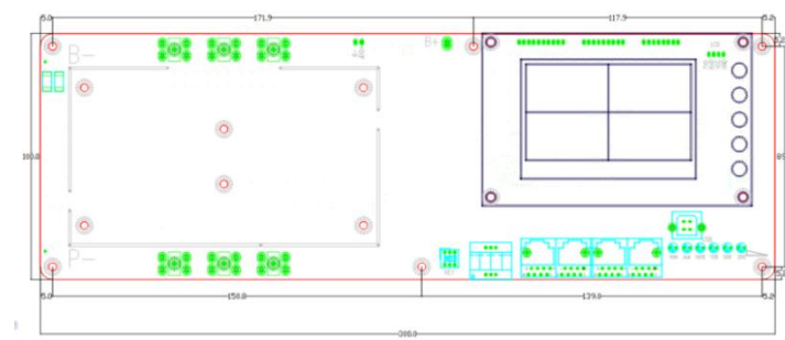
图 10-3 主板尺寸图
