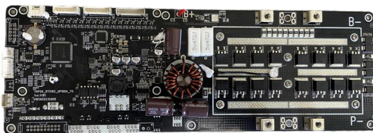
图 10-1 主板标配实物图-正面
