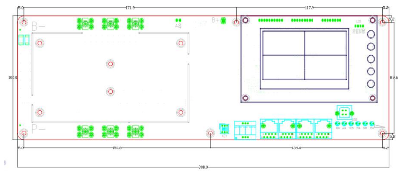
图 10-3 主板尺寸图
