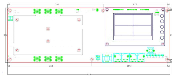
图 10-3 主板尺寸图
