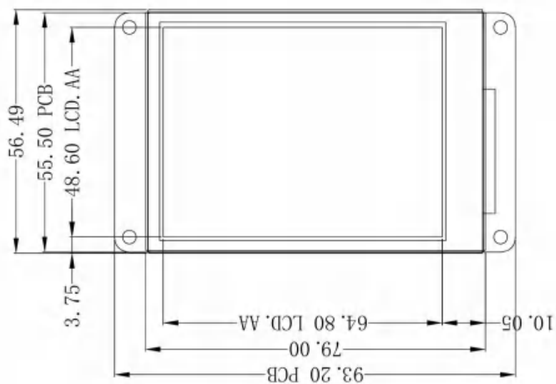
側面尺寸
