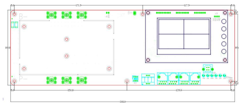
图 10-3 主板尺寸图
