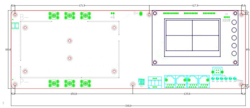
图 10-3 主板尺寸图
