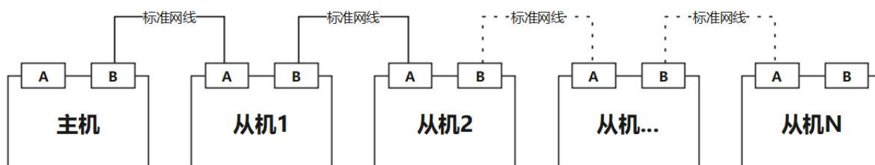
图 8-1 并机接线示意图
