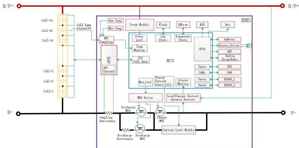
图3-1 功能框图
