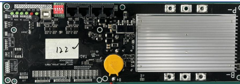
图 10-2 主板标配实物图-反面
