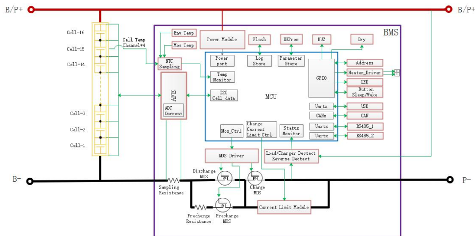
图3-1 功能框图
