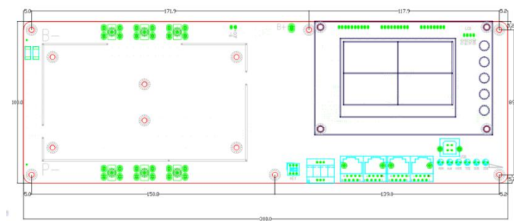
图 10-3 主板尺寸图
