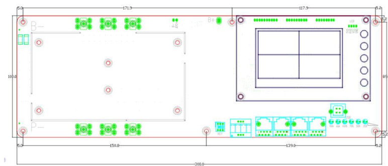
图 10-3 主板尺寸图
